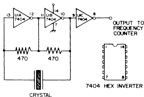
Fig. 4 Hex inverter circuit.
